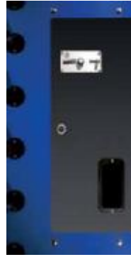
Schublade Nr. 2 vom P4P Soccer Coin-op Mechanischer Münzprüfer mit Ballausgabe. Münzen 0,50 EUR. Optional bestellbar: 1,00 EUR pro Spiel, Währung nach Kundenwunsch.
